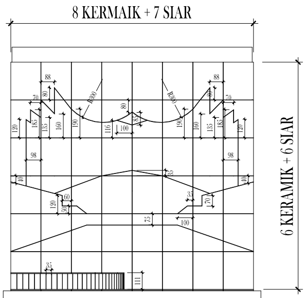
TAMPAK DEPAN
