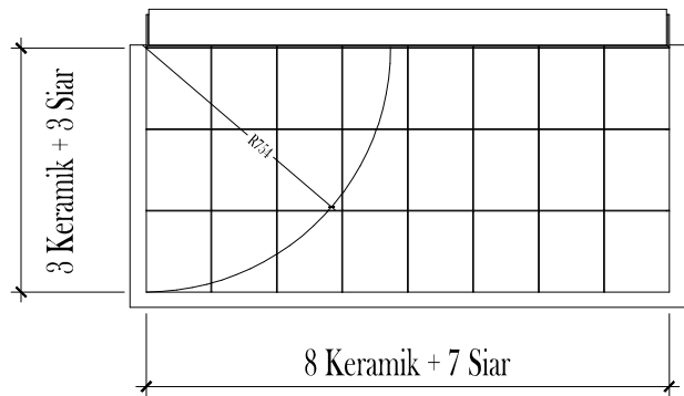
UKURAN LANTAI
