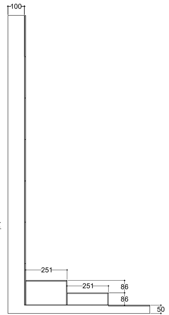
POTONGAN MELINTANG
