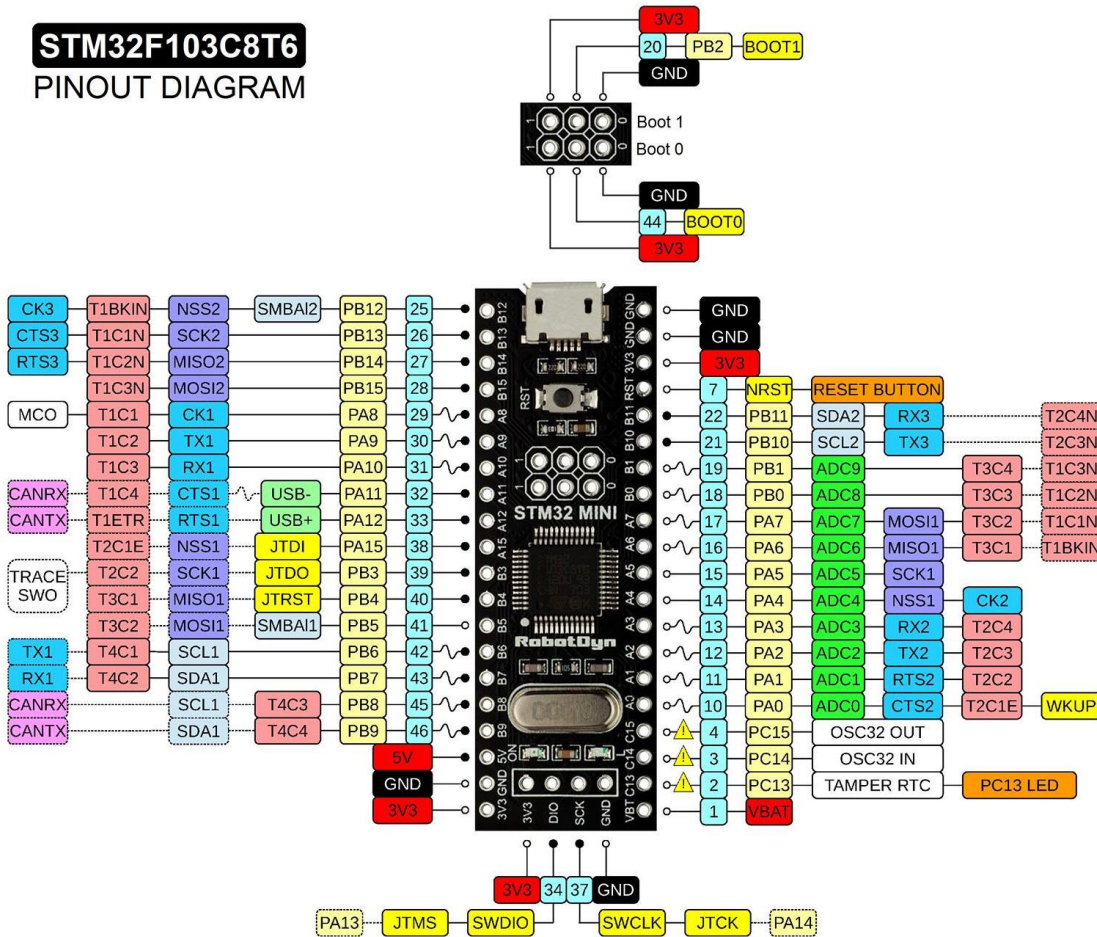
Gambar 2. Konfigurasi I/O MCU
